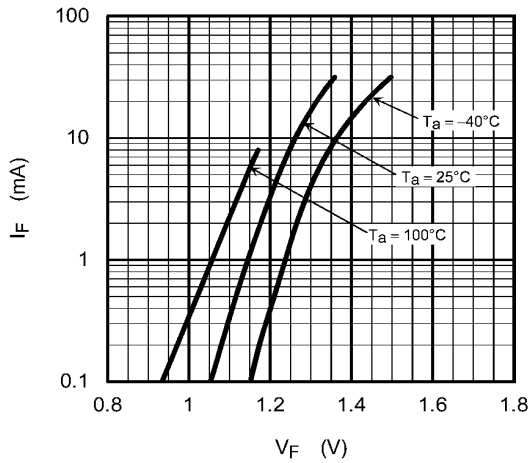
Fig. 11.3 I_F - V_F
