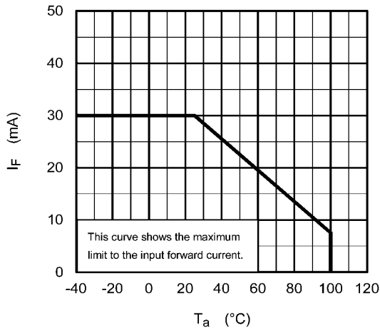
Fig. 11.1 I_F - T_a
